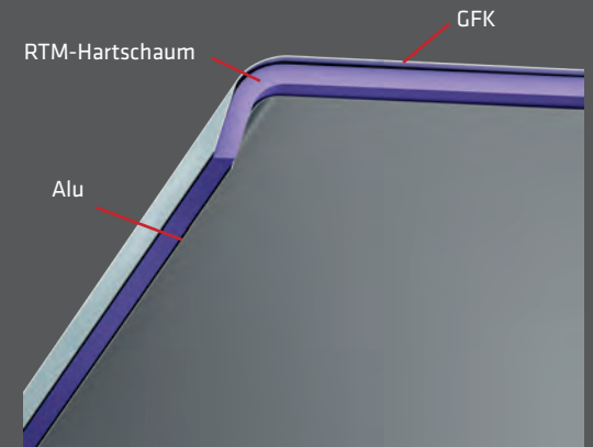
Malibu Van Hybrid-Aufstelldach mit klassenbestem Isolationskonzept in Sandwichbauweise und mit geringem Eigengewicht
